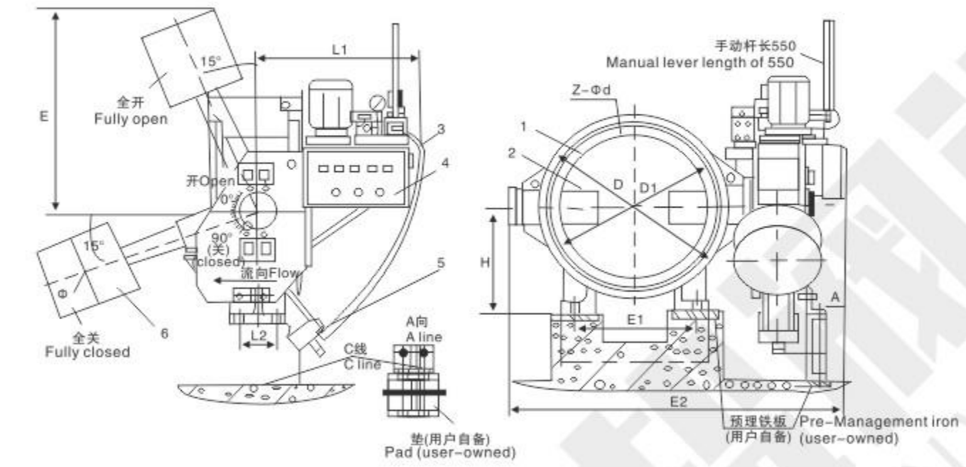
1、阀体 2、蝶板 3、液控系统 4、电控箱 5、摆动油缸 6、重锤 1, Body 2, disc 3, hydraulic control system 4, electric control box 5, swing cylinder 6, hammer 正装型 Dress Type
