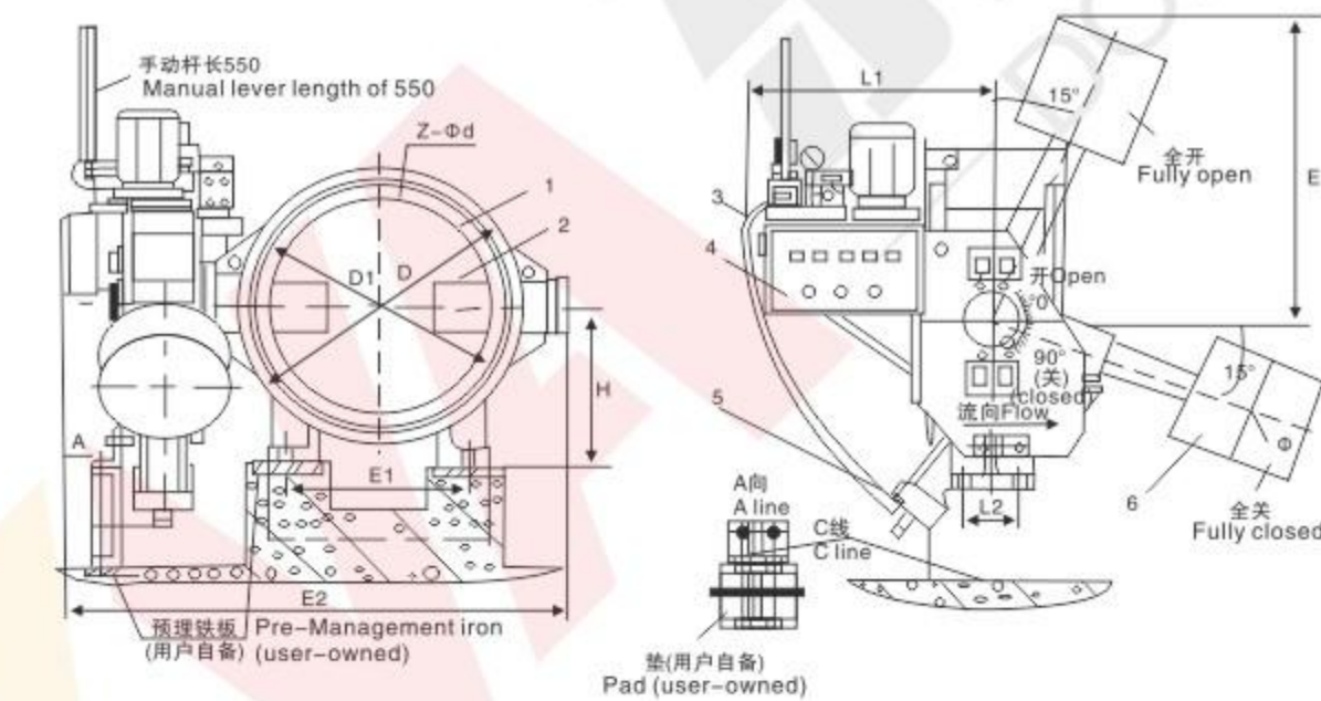
1、阀体 2、蝶板 3、液控系统 4、电控箱 5、摆动油缸 6、重锤 1, Body 2, disc 3, hydraulic control system 4, electric control box 5, swing cylinder 6, hammer 反装型 Anti-mounted type
