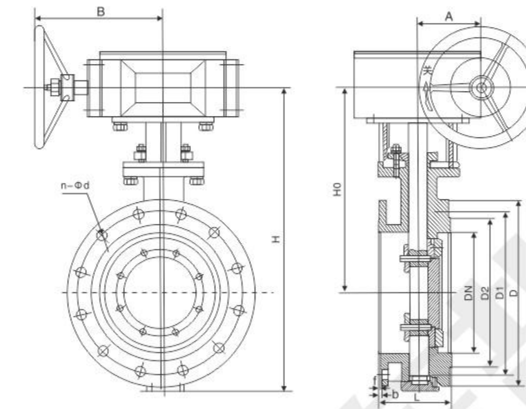
主要连接尺寸 Main connection dimensions
