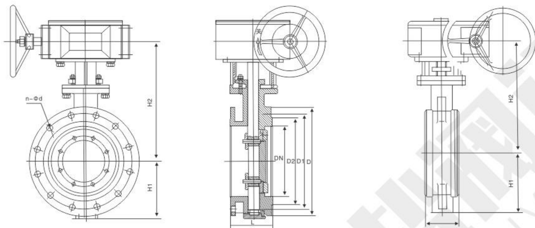
主要连接尺寸 Main connection dimensions
