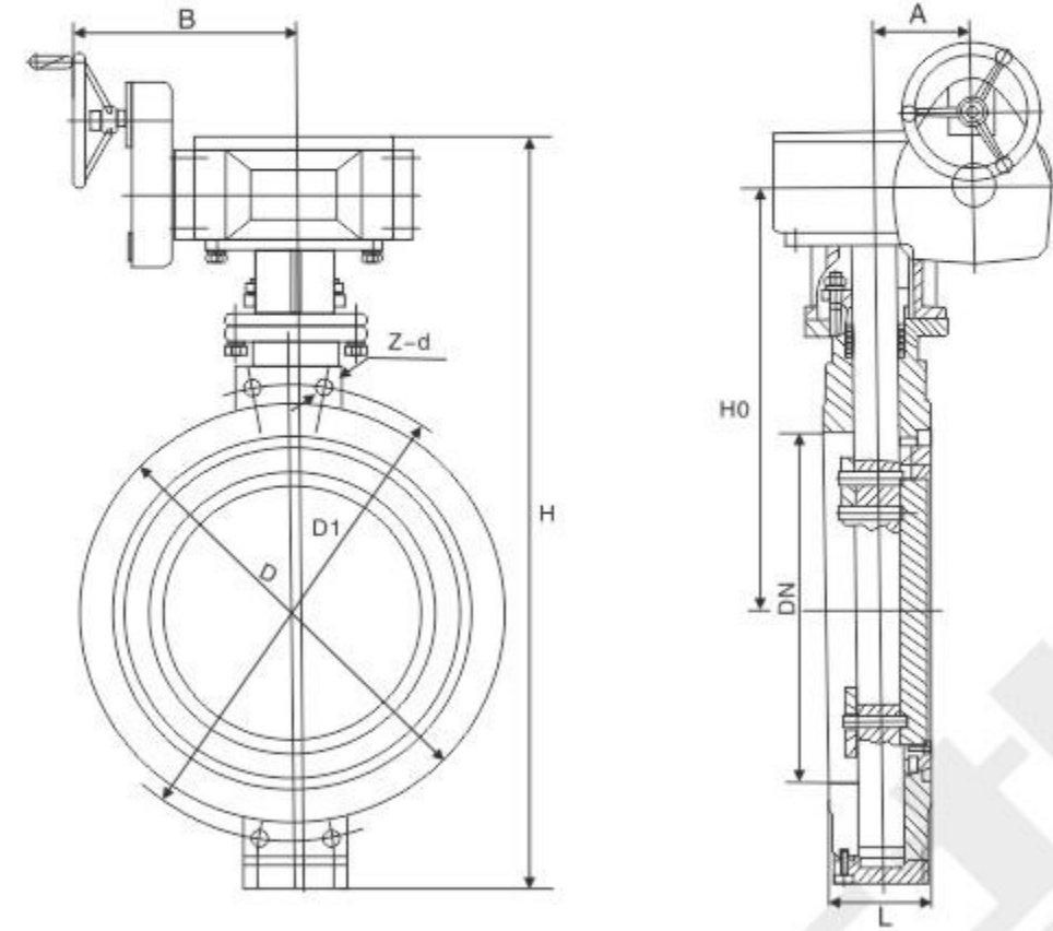
主要连接尺寸 Main connection dimensions
