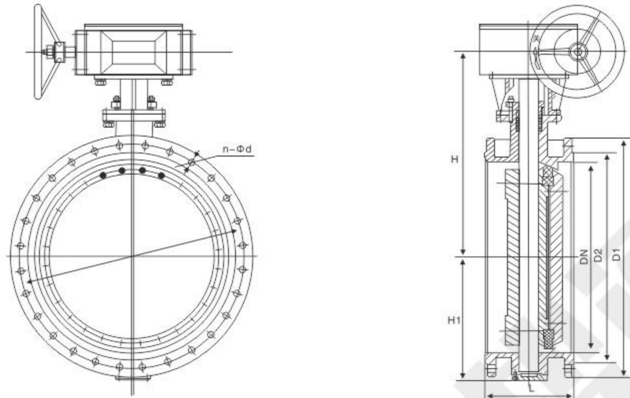
主要连接尺寸 Main connection dimensions
