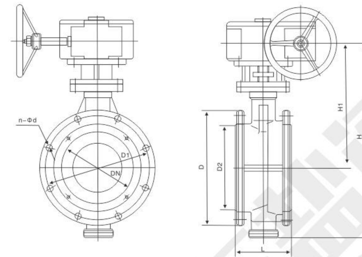
主要连接尺寸 Main connection dimensions
