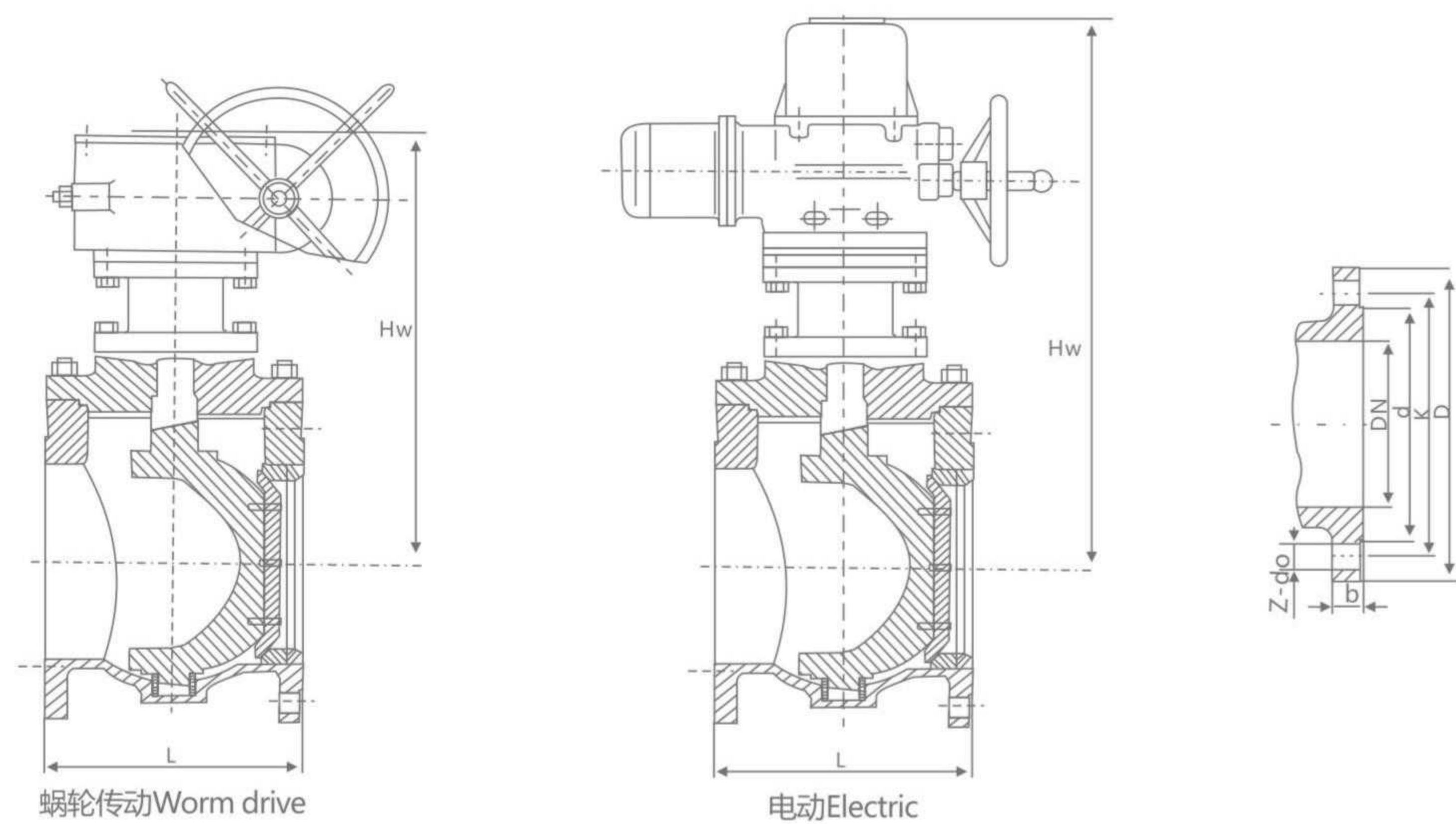
主要连接尺寸 Main connection dimensions
