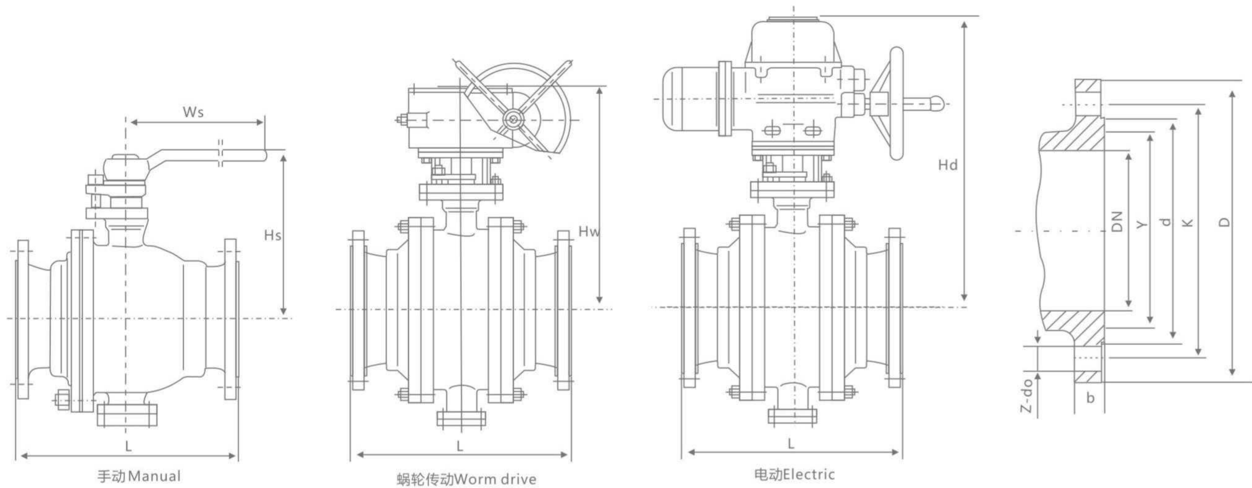
主要连接尺寸 Main connection dimensions JB/T79.1
