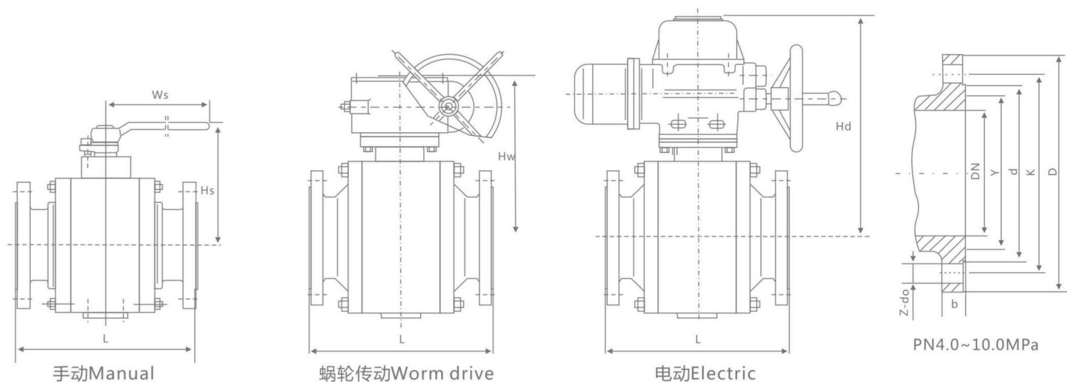
主要连接尺寸 Main connection dimensions
