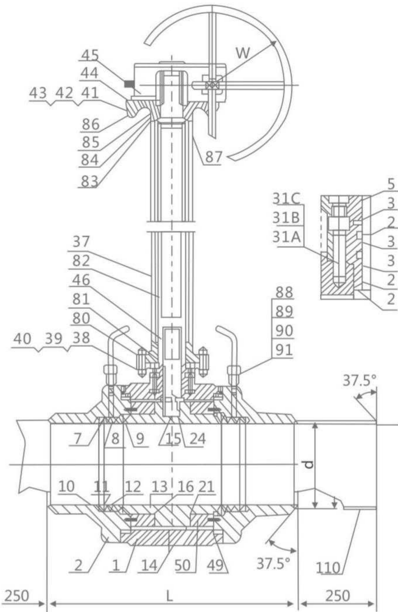
结构图Structure diagram
