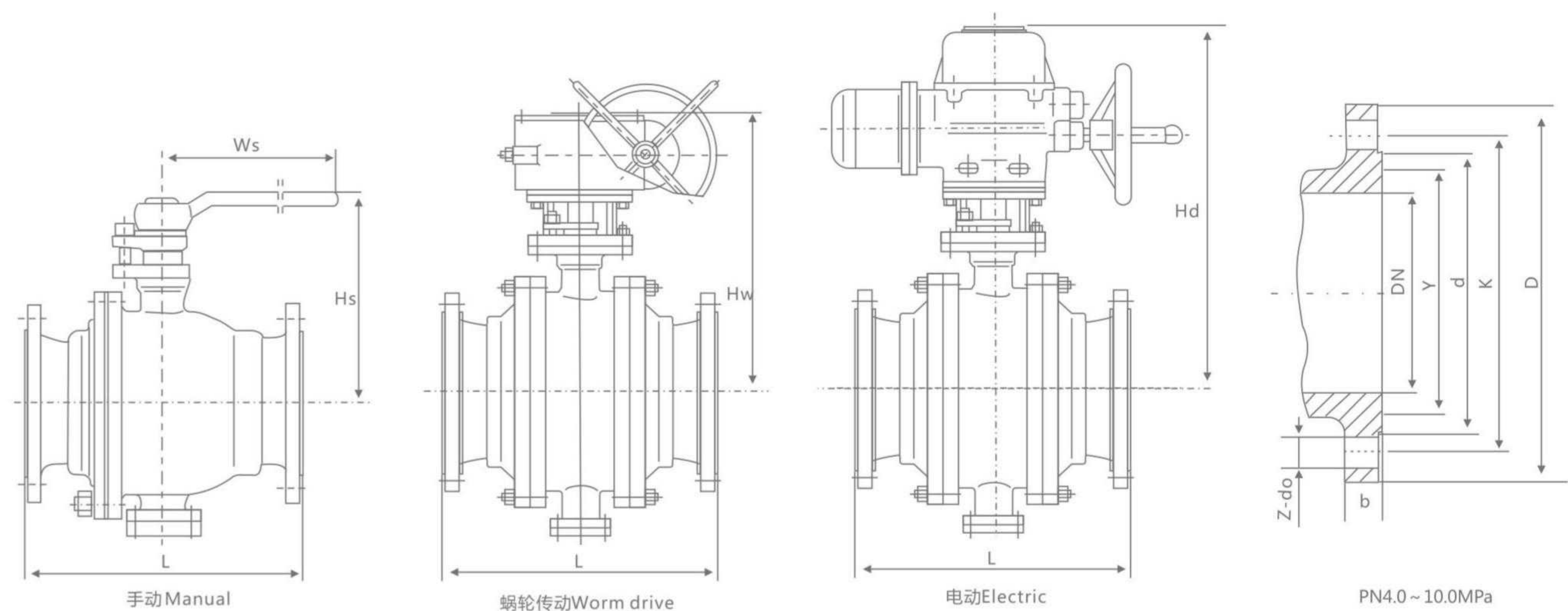
主要连接尺寸 Main connection dimensions
