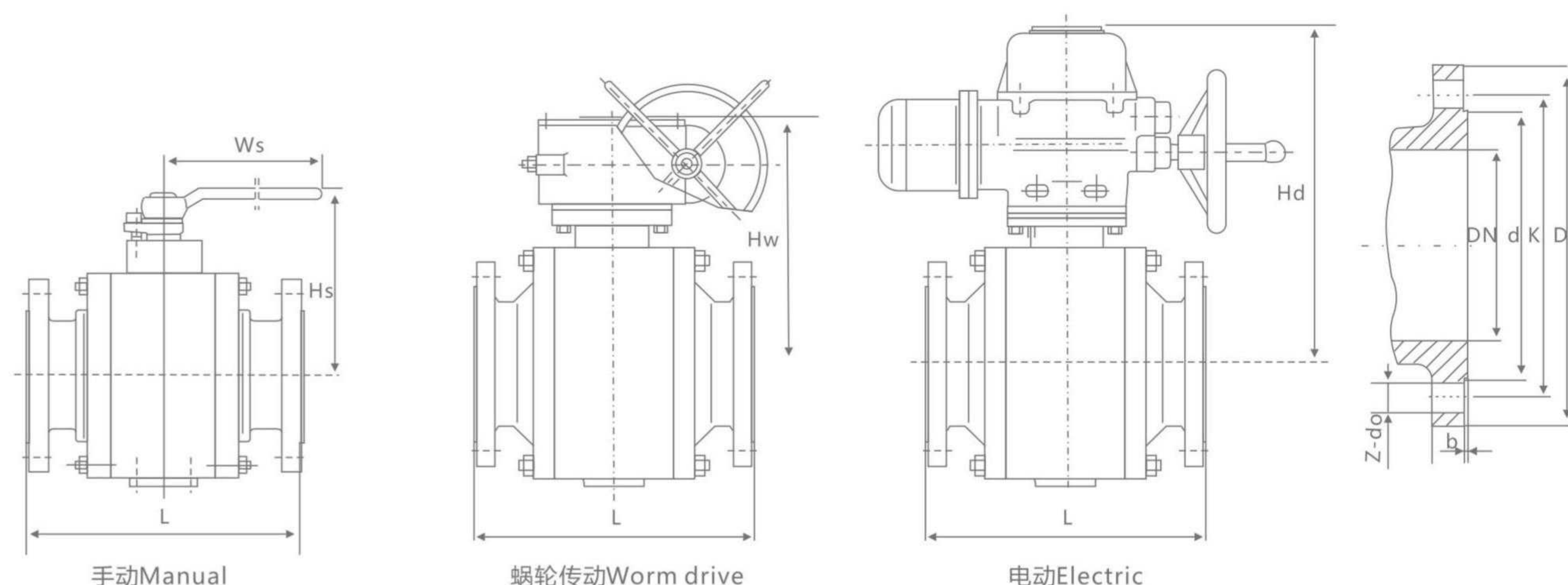
主要连接尺寸 Main connection dimensions
