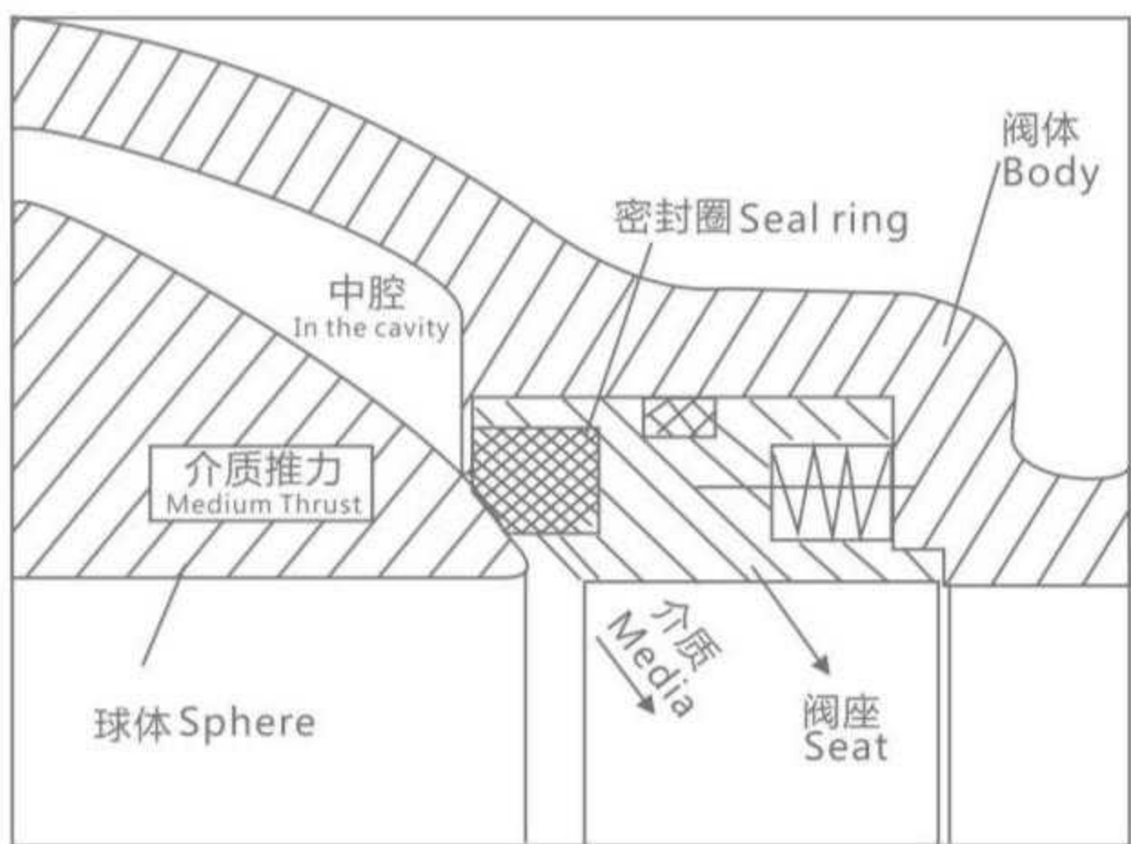
自动卸压功能 Automatic pressure relief feature
